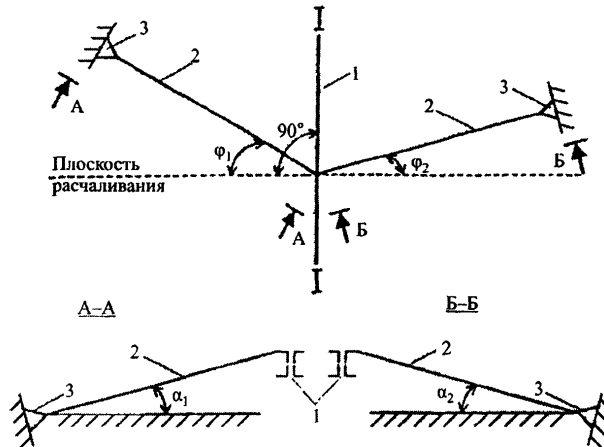
1 – ферма; 2 – расчалка; 3 – якорь
